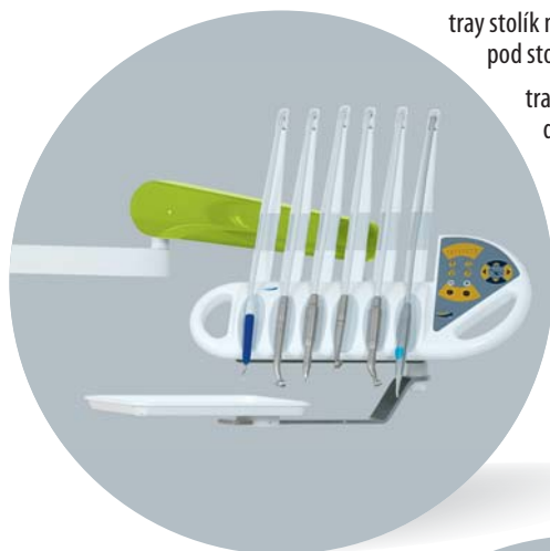
трей-столік на удлиненом плече под столиком врача
